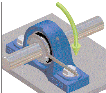
4. Sicherungsblech und Nutmutter montieren und anschließend mit empfohlenen Anzugsmoment anziehen.
