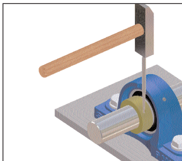
4. Excenterring mit Dorn und Hammer festspannen.
